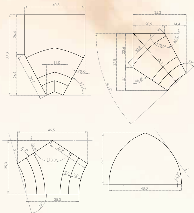
Les plans d'exécution par l'entreprise Fabien Michel
