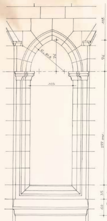
Les relevés de l'architecte Robert Falarz
